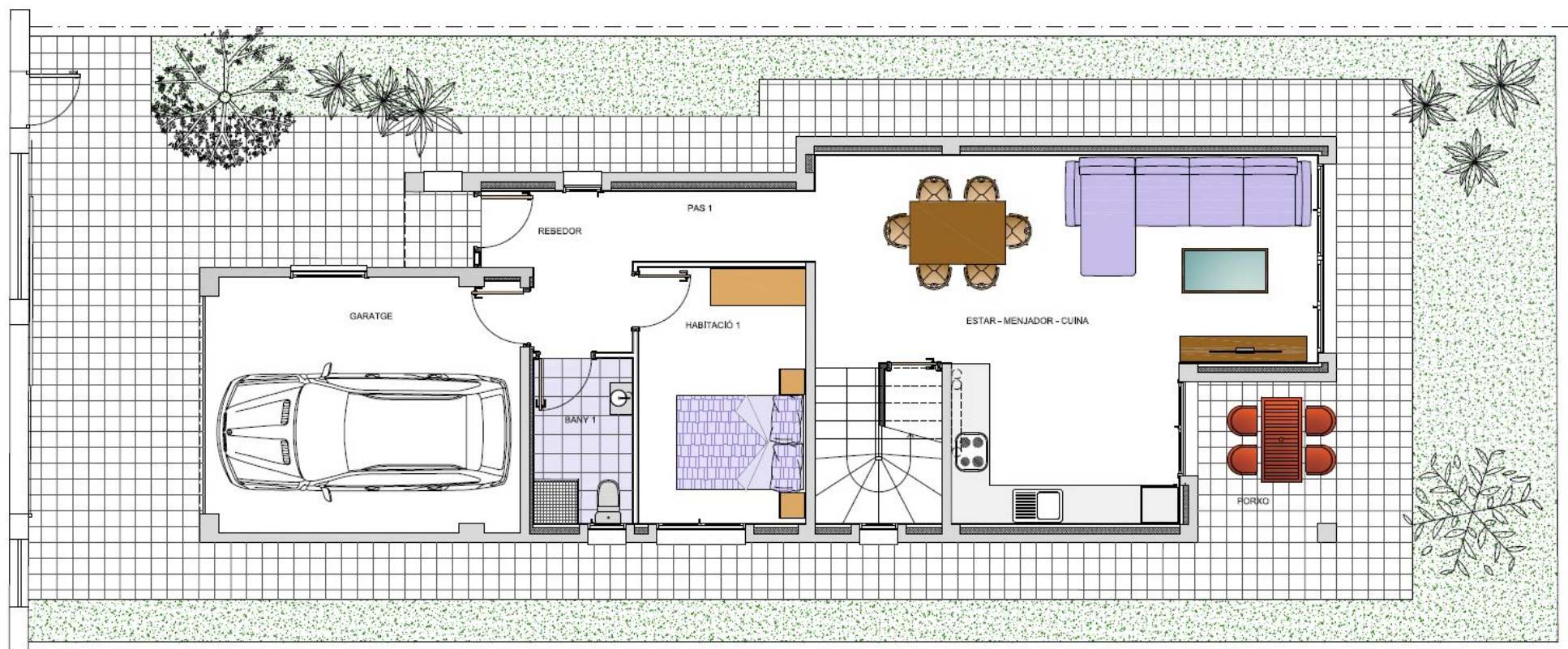
PLANTA BAIXA
